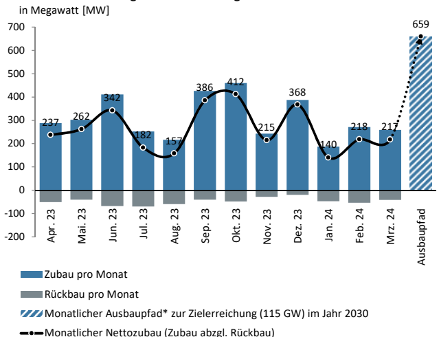
Monatlicher Leistungszubau Windenergie an Land
